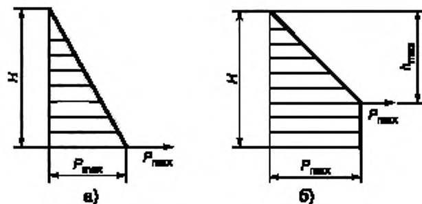
Рисунок Д.1— Расчетные эпюры бокового давления бетонной смеси
